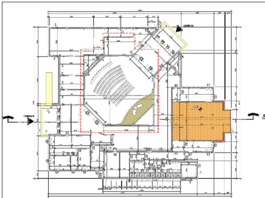
1 PIANTA QUOTA 0,00 scala 1:200
