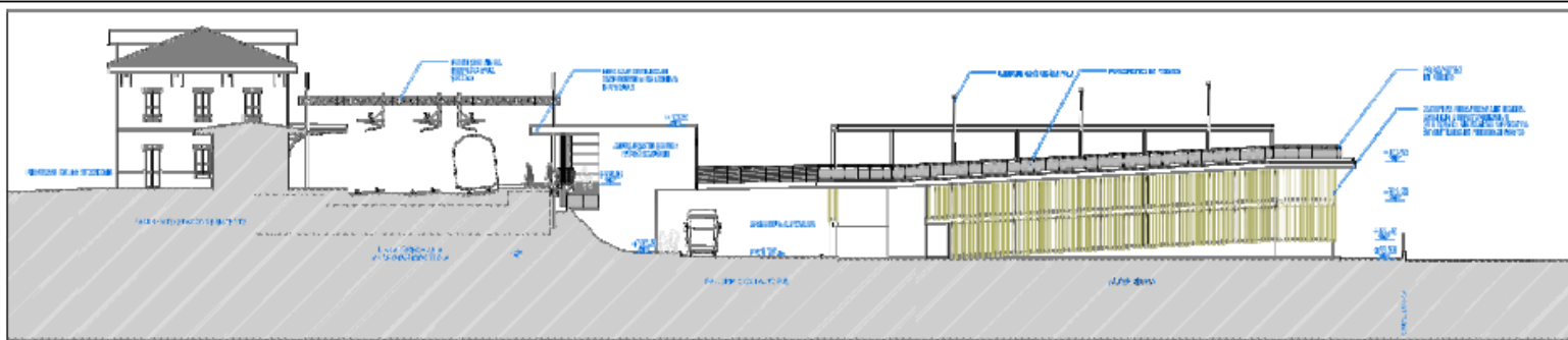
1 PROSPETTO SUD Elev. 1/200
