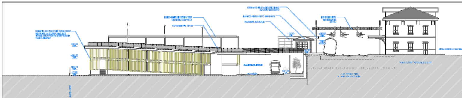
3 PROSPETTO NORD Elev. 1/200
