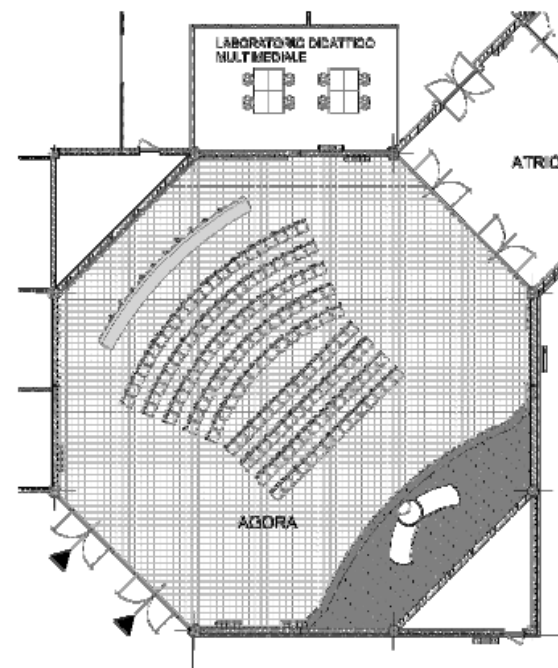
2 PIANTA QUOTA 0,00 CON INDICAZIONE LOCALI scala 1:500
